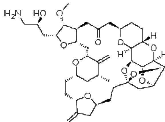
Eribulin
