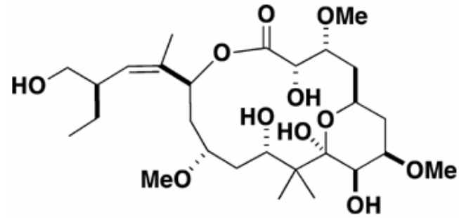
Peloruside
