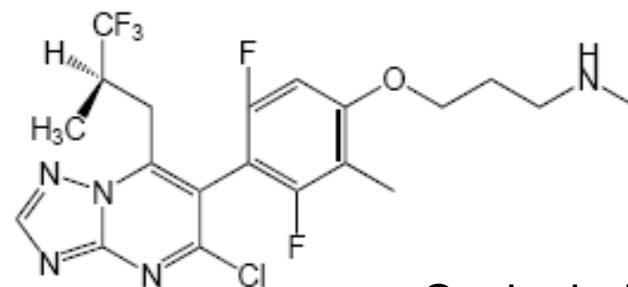
Cevipabulin
