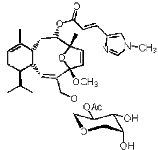
Eleutherobin
