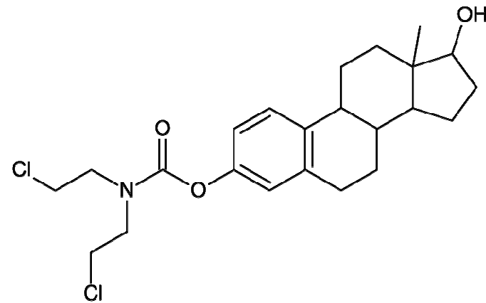
Estramustine
