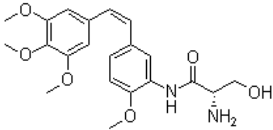
Ombrabulin
