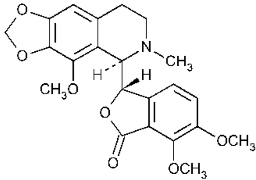
Noscapine
