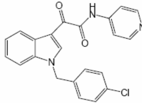
Indibulin
