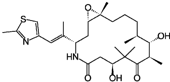
Ixabepilone
