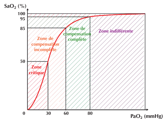
Figure 2. Courbe de tolérance à l'hypoxie (d'après Strughold, 1954). SaO 2 : saturation du sang en oxygène, PaO 2 : pression partielle d'oxygène dans le sang artériel.
